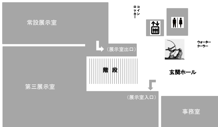
美術館1階平面図
